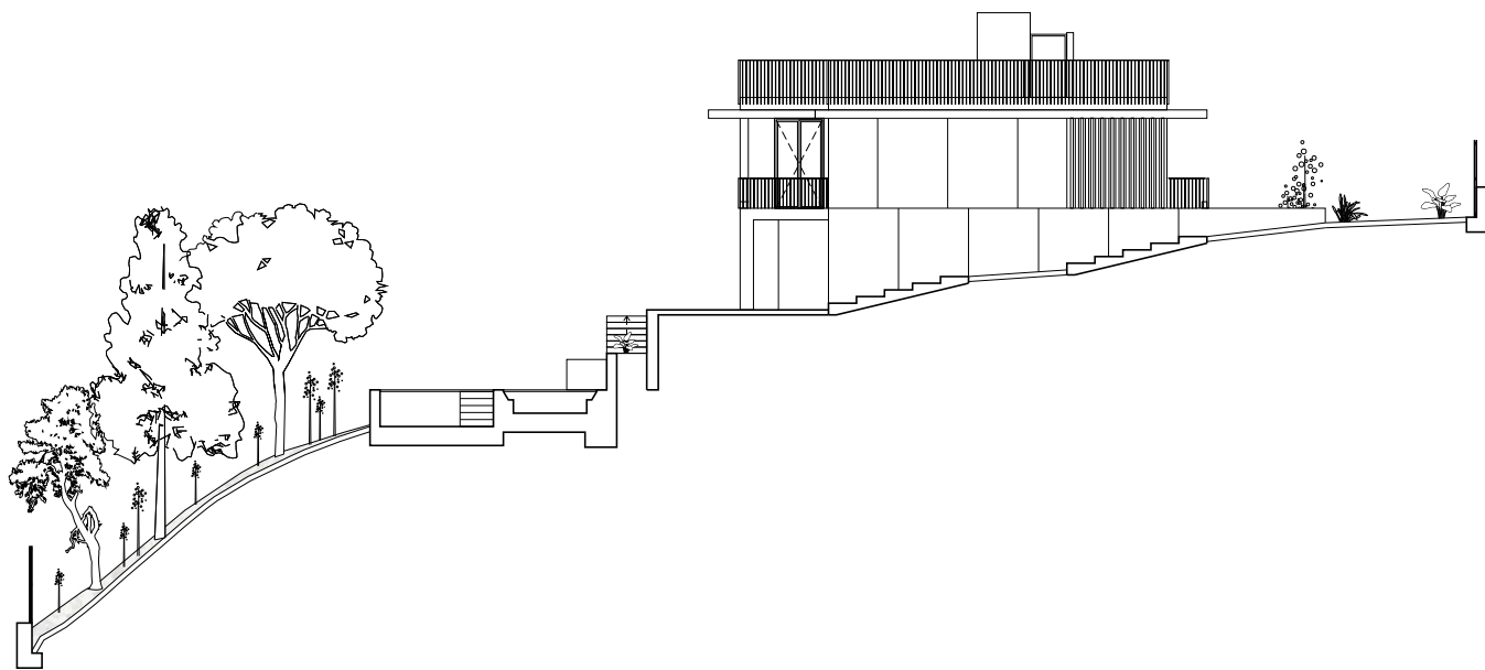
Alzado Este
