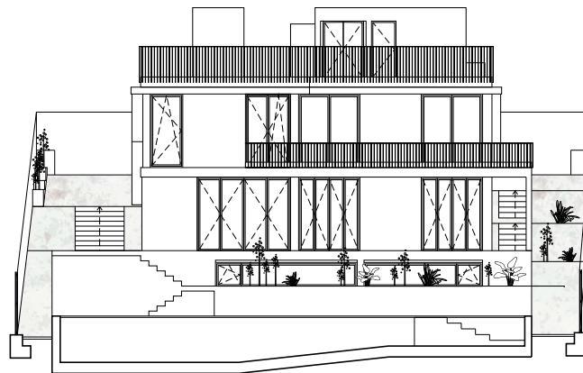
Alzado Sur
