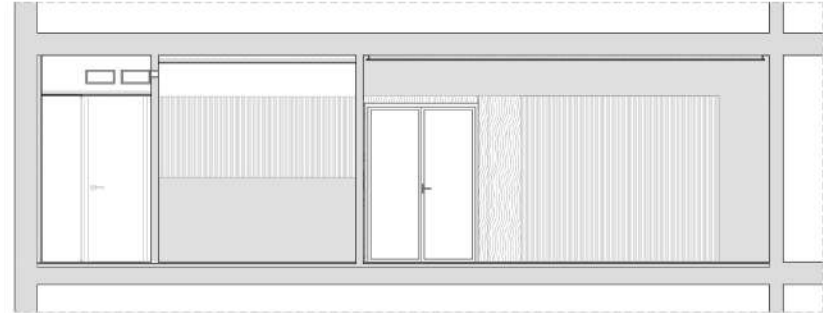
SECCIÓN C-C' ESTADO REFORMADO
