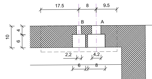
DETALLE AGUJEROS GRIFO Y MANDO
