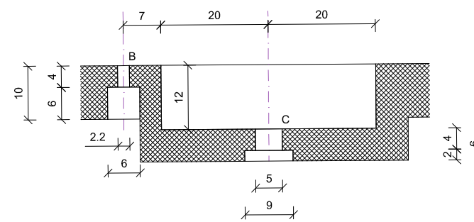
DETALLE AGUJEROS DESAGUE Y GRIFO
