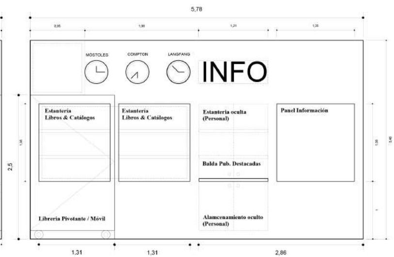
Alzado Frontal (Zona Lobby)
